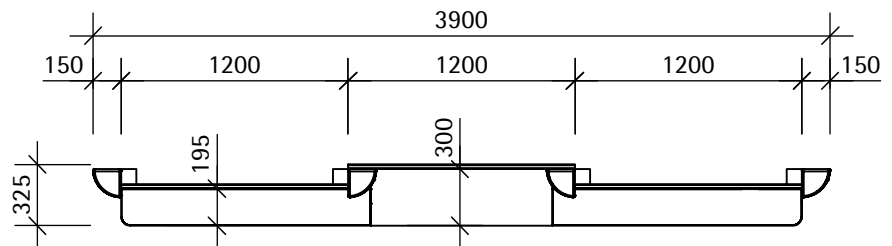
DRAUFSICHT
