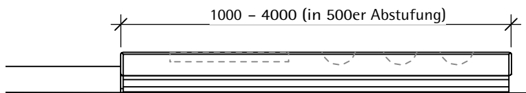
VORDERANSICHT
