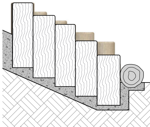
SCHNITT
