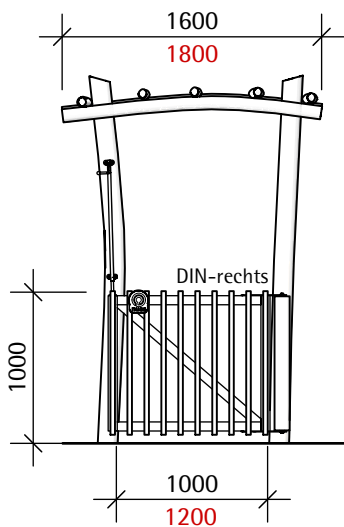
VORDERANSICHT
